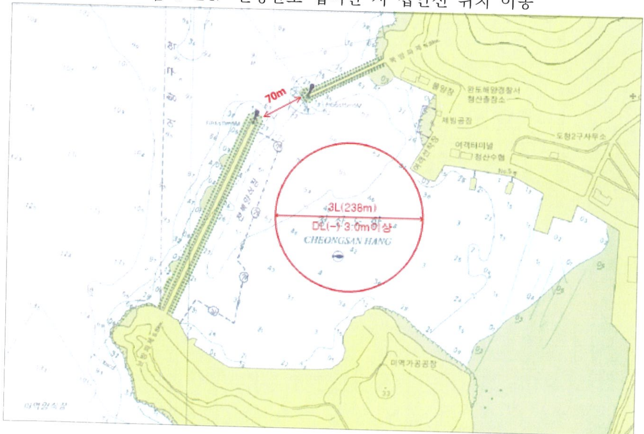
<그림 5-25> 킨청산호 출항 시 선회수역 확보
